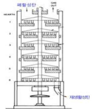
[다단로 재생공정]
