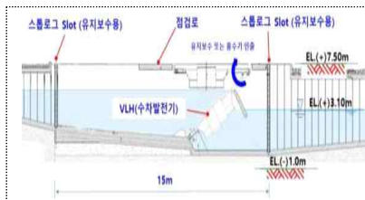
잠실수중보 설치 예상도
