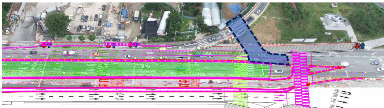
[그림 5] 사업대상지 공사 중첩구간 현황
