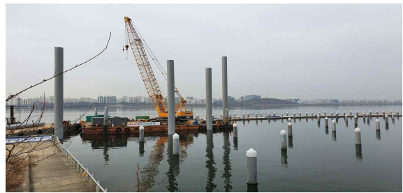
텔레스코프 파일, 부방파제 설치
