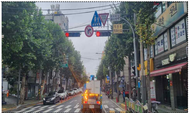
〔교체 전〕 마포구 성산초교 교차로 차량신호 모듈 교체 〔교체 후〕
