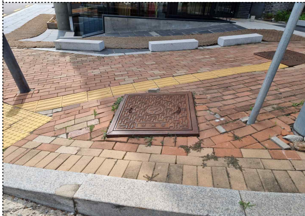
〔단차 조정 전〕 은평구 하나고 앞 신호맨홀 단차 〔단차 조정 후〕
