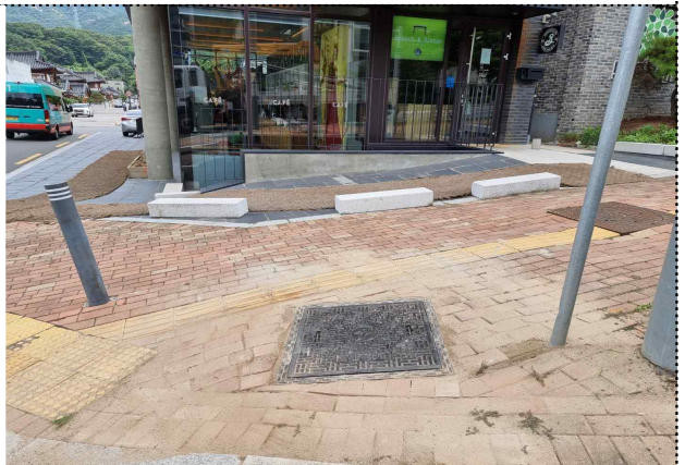
〔단차 조정 전〕 은평구 하나고 앞 신호맨홀 단차 〔단차 조정 후〕
